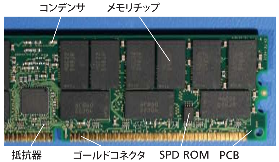
メモリモジュールの主要部位
